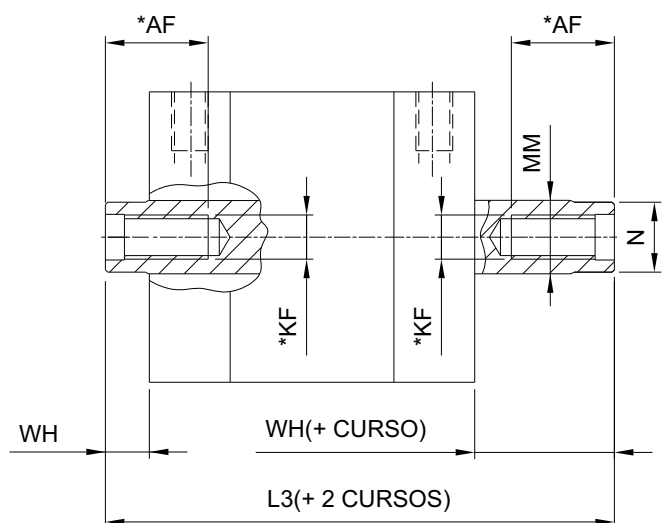
Haste Passante com Rosca Fêmea
