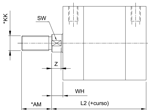
Haste com Rosca Macho
