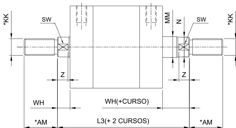
Haste Passante com Rosca Macho
